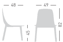
ALHAMBRA BL Technopolimer padded and upholstered shell. Beech wooden frame Scocca in tecnopolimero, imbottita e rivestita. Telaio in legno.
