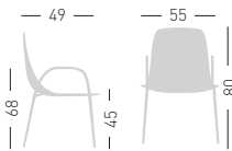
COLORFIVE TB Techno polymer upholstered shell, chromed or painted metal frame with arms. Scocca in tecnopolimero rivestita, telaio in metallo cromato o verniciato con braccioli.
