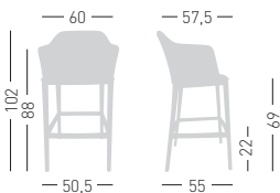
MANAA 69 Upholstered barstool, techno polymer base. Sgabello rivestito, telaio in tecnopolimero.
