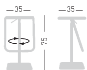
JOE Wooden beech seat, base and frame in chromed metal. Seduta in legno di faggio, telaio e base in metallo cromato.
